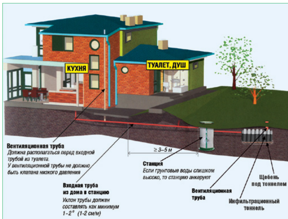
Рис. 2 Схема установки станции FloTank-BioPurit
