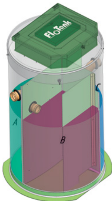
Рис. 1 Схема станции FloTank-BioPurit
